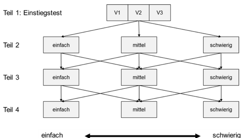
Abbildung 1: Aufbau der adaptiven Online-Tests
